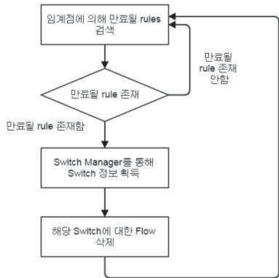
그림 4. 공격 방어기의 룰 삭제 알고리즘
