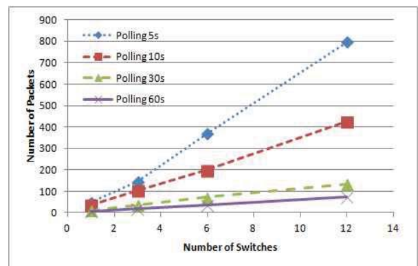
그림 10. Polling과 스위치 개수에 따른 샘플 패킷량
