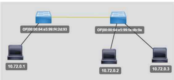
그림 6 로컬 테스트베드 네트워크 구성도
