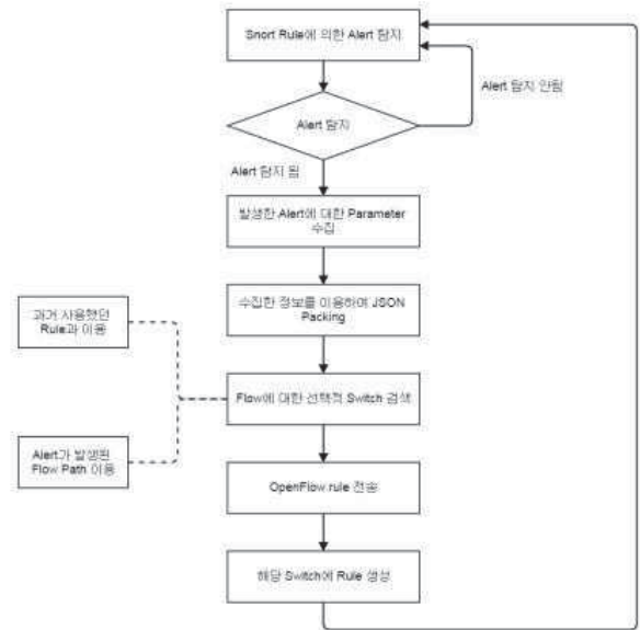
그림 3. 공격 방어기의 룰 생성 알고리즘
