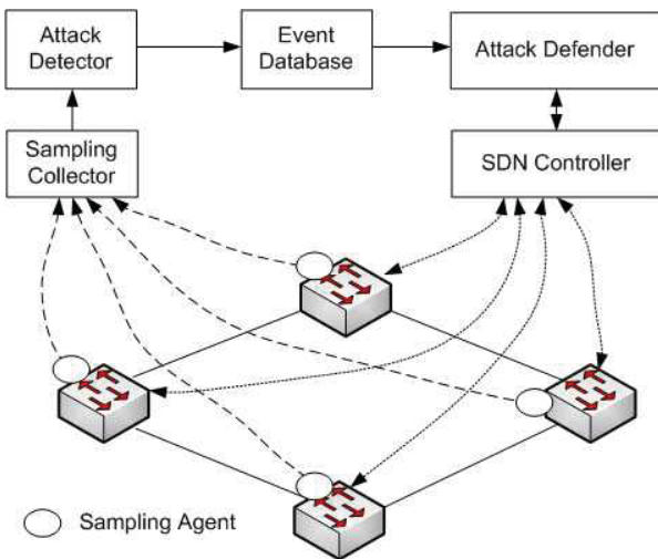
그림 2. 샘플링 기반 공격 탐지 방어 시스템 구조
