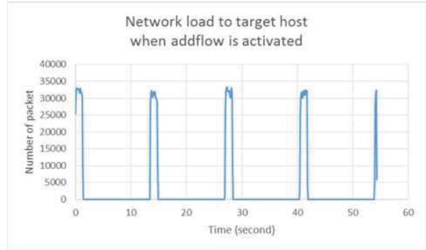
그림 8. 공격대상 호스트 네트워크 트래픽
