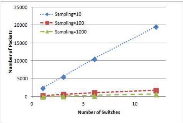
그림 9. Sampling Rate와 스위치 개수에 따른 샘플 패킷량
